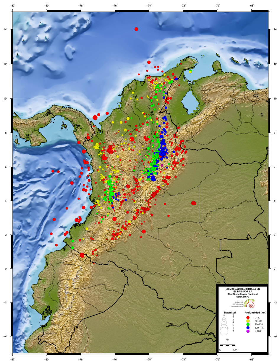
Figura 3.6. Eventos durante octubre de 2023
