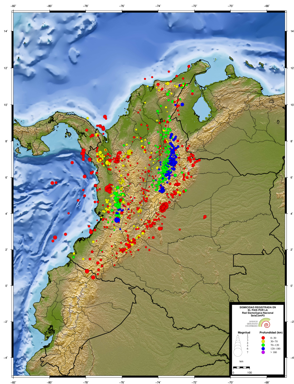
Figura 3.4. Eventos durante agosto de 2023
