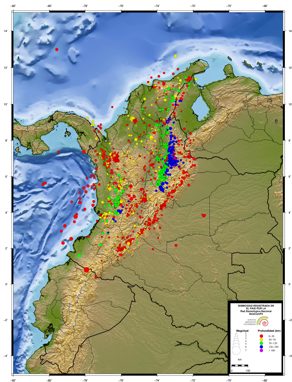
Figura 3.8. Eventos durante diciembre de 2023
