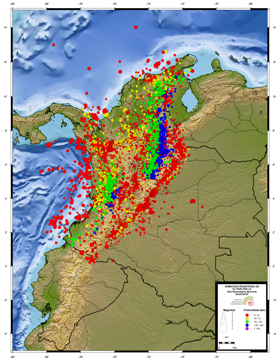
Figura 3.2. Eventos localizados por el SGC durante julio-diciembre de 2023
