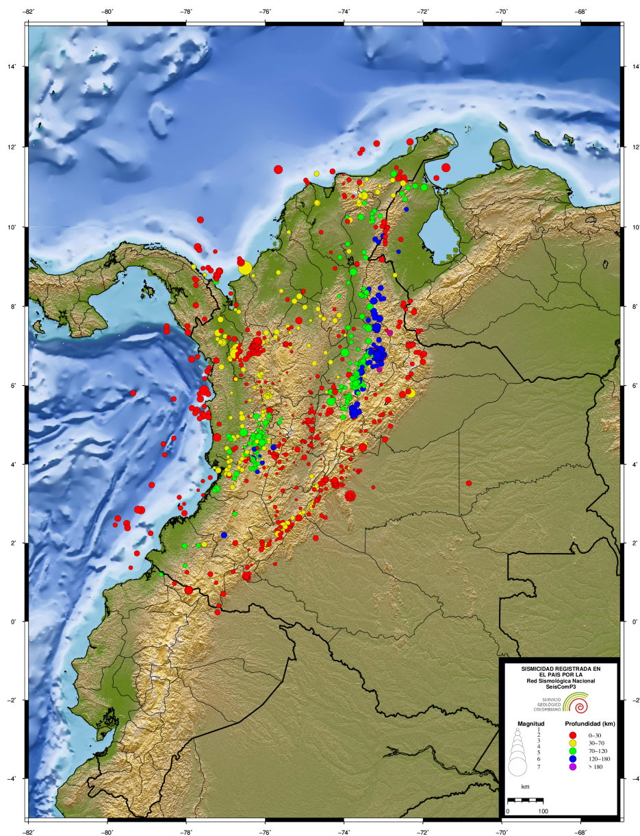
Figura 3.3. Eventos durante julio de 2023
