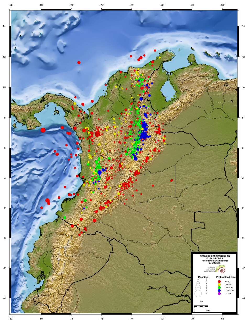
Figura 3.7. Eventos durante noviembre de 2023
