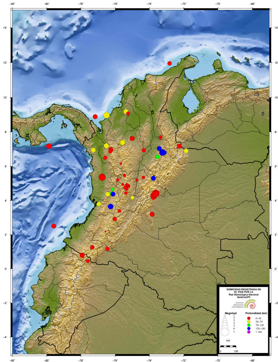
Figura 3.1. Sismos destacados localizados por el SGC durante julio-diciembre de 2023
