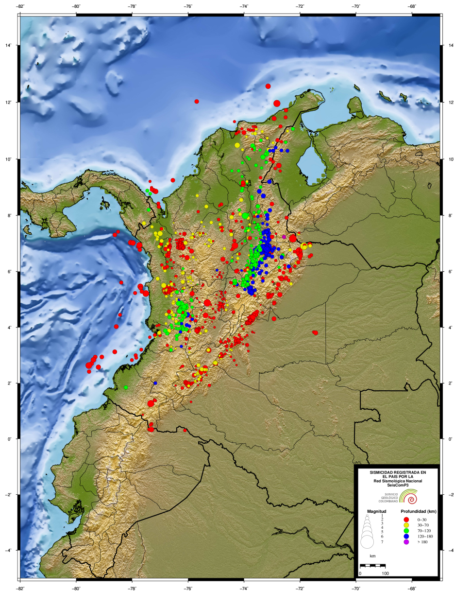
Figura 3.5. Eventos durante septiembre de 2023
